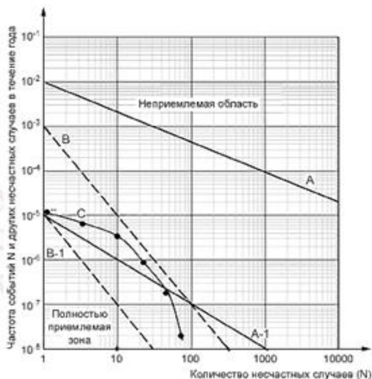
Рисунок Б.15 — Пример диаграммы F-N
