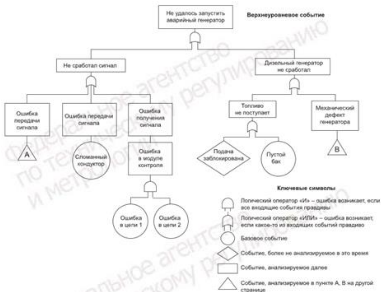
Рисунок Б.5 — Пример дерева отказов
