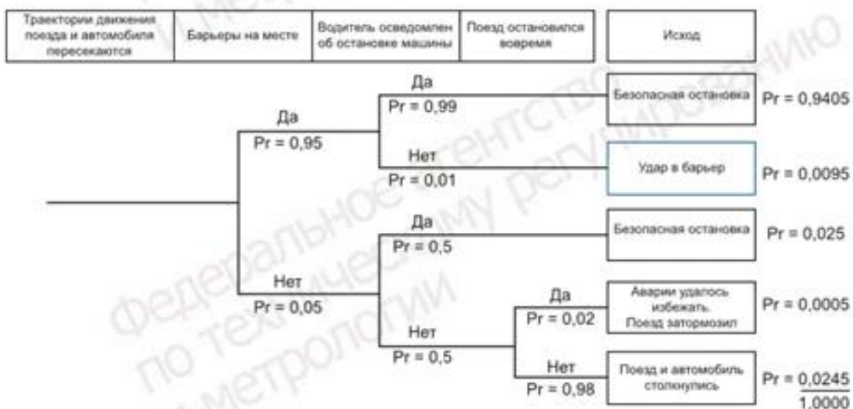
Рисунок Б.4 — Пример анализа дерева событий
